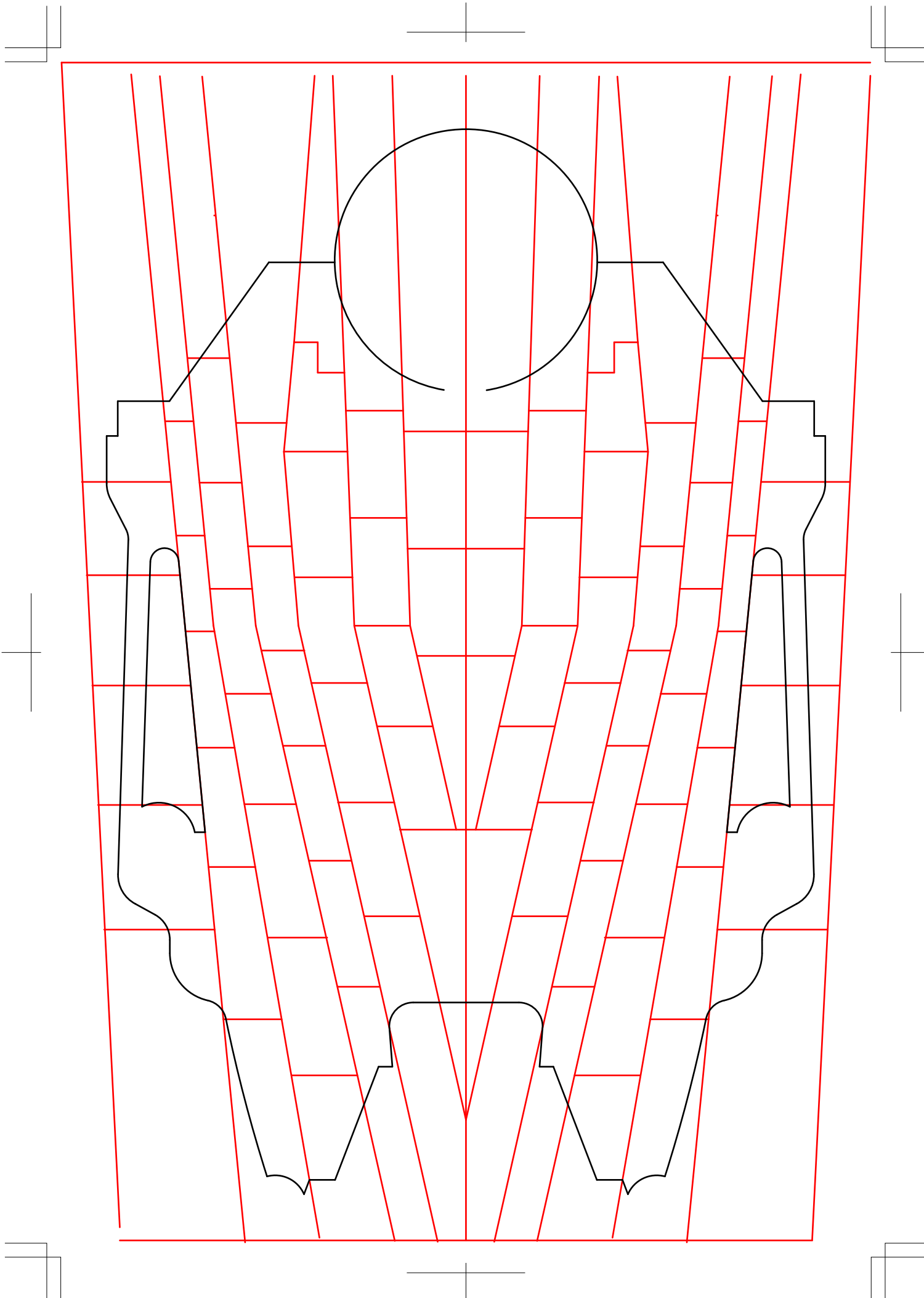
1:250 戦艦大和 (レール甲板とタイル模様)
